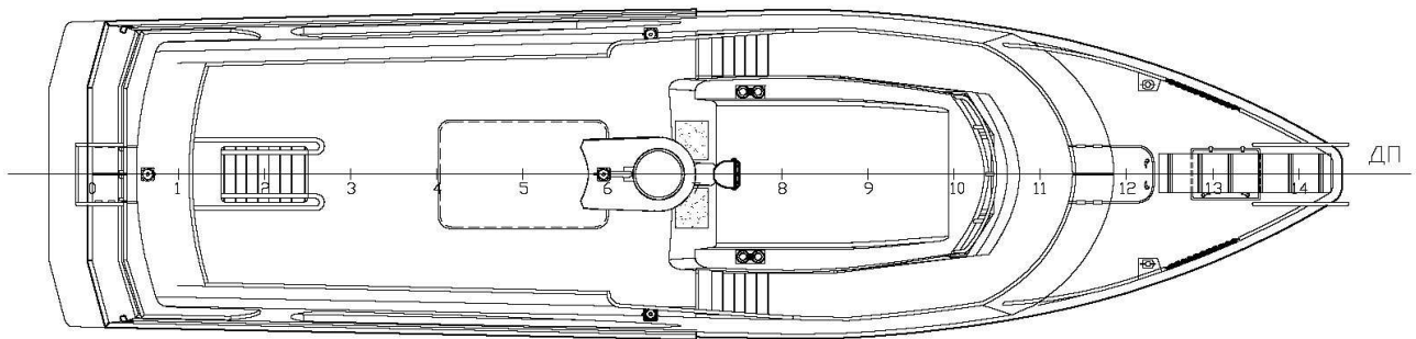
Верхняя палуба
