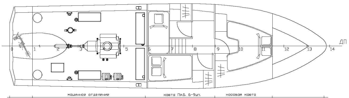
ТРЮМ
